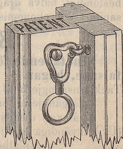
Concenterisk haspe till vanl. utg. fönster.
