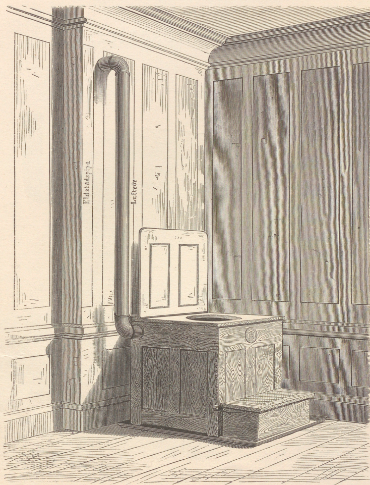
Garderobs-klosett, utvisande lufrörets uppsättning.
