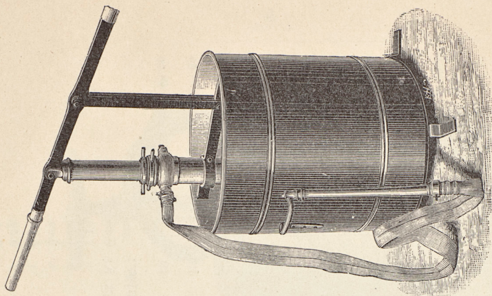
N:o 13, Länsspruta.
