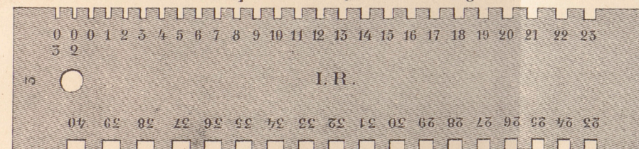
Mått för superfina cylinder-urfjedrar.
