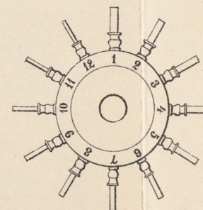
Mått för nyckelrör.
