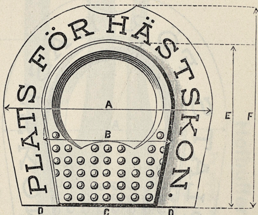
Dimensioner i mm. å Gummi-Hästskor för framfötter. fig. 12.
