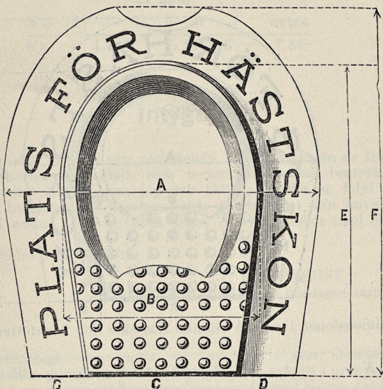
Dimensioner i mm. å Gummi-Hästerskor för bakfötter, fig. 11.
