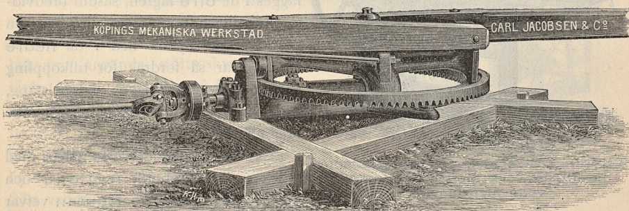
Köpings liggande vandring n:o 17, för 1 å 2 dragare.
