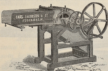
Köpings Stiftröskverk N:o 3 såsom handtröskverk med hufvudaxeln i de öfre lagren.
