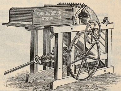
Köpings Stifttröskverk N:o 4 och N:o 7 med ändutvexling och dubbla par lager.
