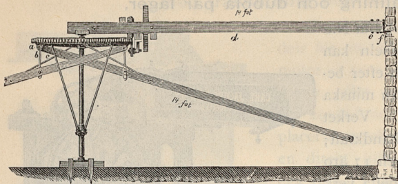
Köpings stående vandringar N:o 10 och N:o 12.
