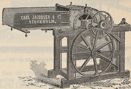
Köpings Stifttröskverk N:o 3 och N:o 6 med hufvudaxeln nedflyttad i de nedre lagren för direkt tillkoppling till vandringsarne.
