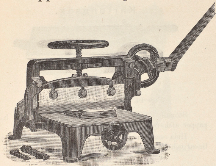
Fig. 13. Pappersskärningsmaskin N:o 1. Skärlängd 12 v. t.
