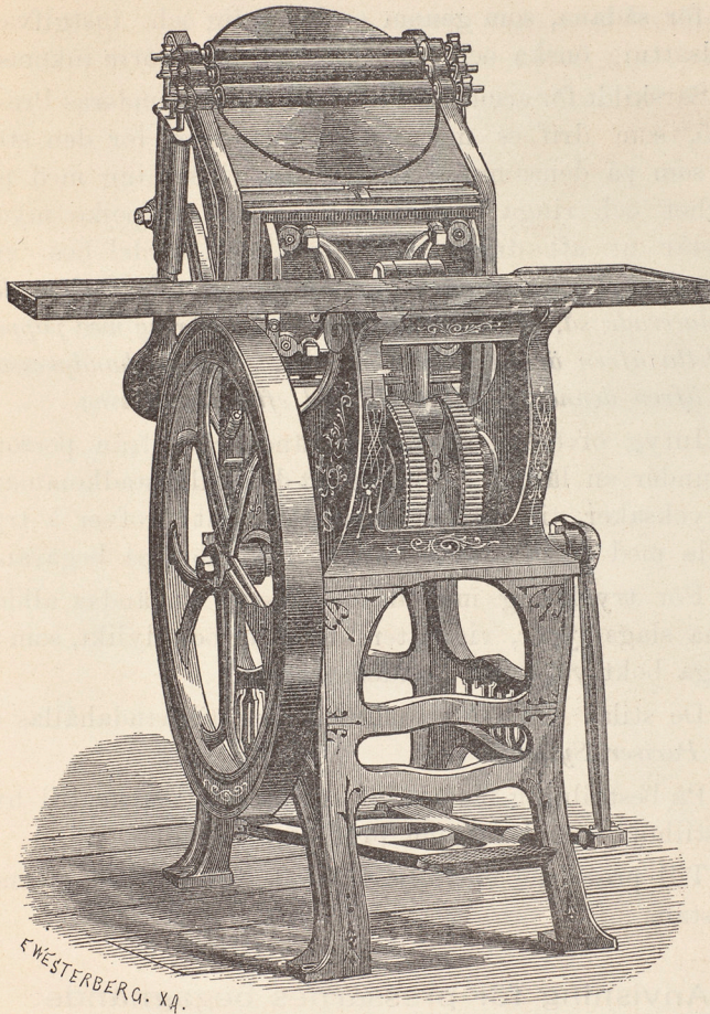
Fig. 4. Sjelffärgande Modell-Snällpress N:r 5.
