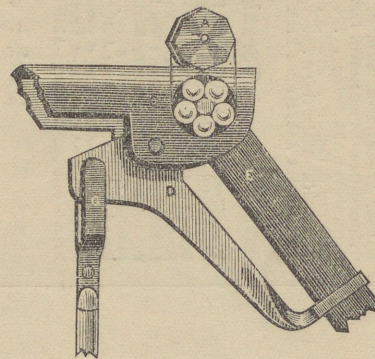
Ofvanstående illustration visar typarmslagret med lagerskålen aftagen, så att axeln och kulorna tydligt synas.
