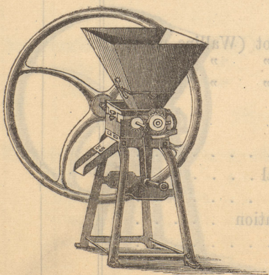
Sädes-kros-maschin.
