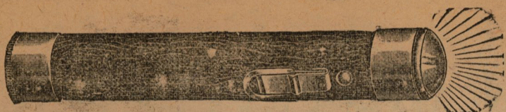
L 60. Elektrisk cylinderlampa , extra stor och ljuskraftig. 230×35 mm. Kompl. pr st. kr. 2.—. Extra Export-batteri, 180×30 mm. Pris pr st. 80 öre.
