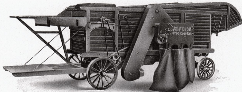
Nya Reform-Tröskverket II A. Transportabelt.
