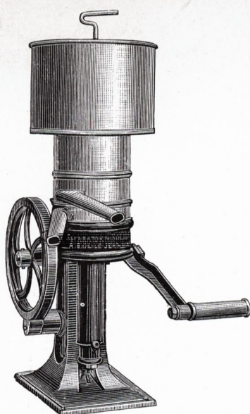
The Separator FLORA.
