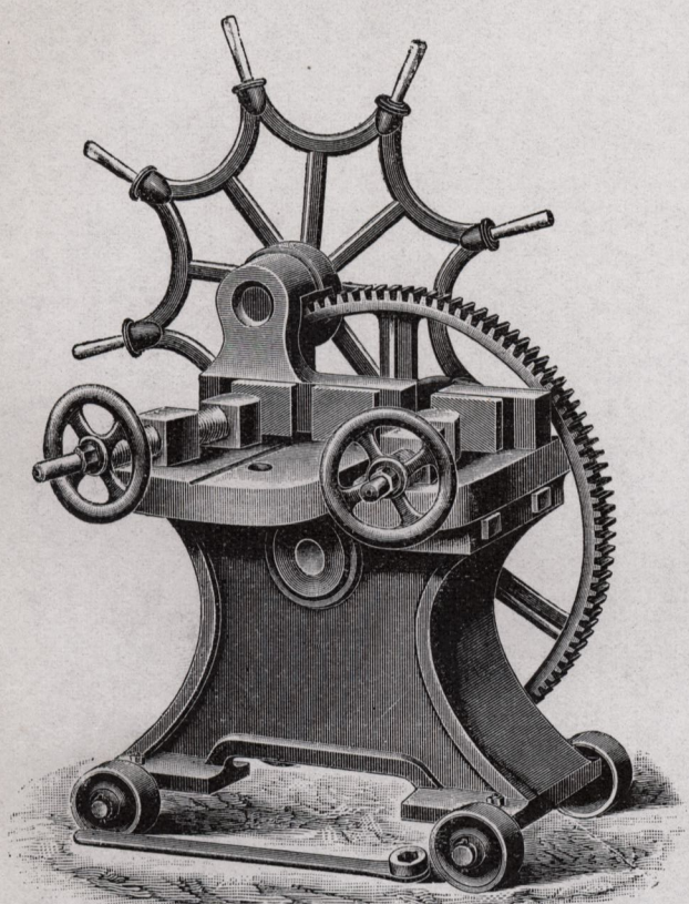
N:r 1 a och 1 b med enkellagrade klämbäckar och dubbellagrad vefaxel.
