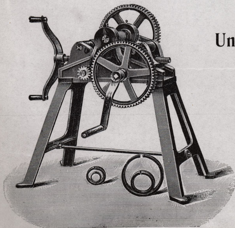
N:r 1 a och 1 b med enkellagrade klämbäckar och dubbellagrad vefaxel.
