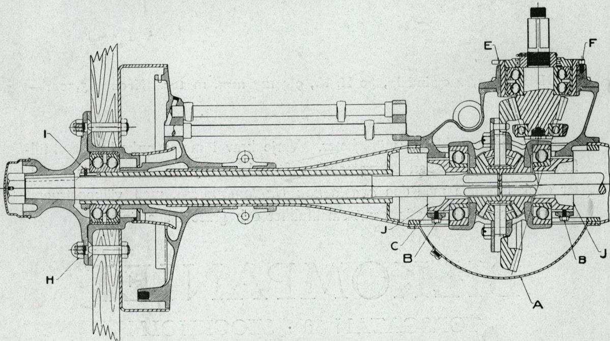
Oaklands differential och »full floating» bakaxel
