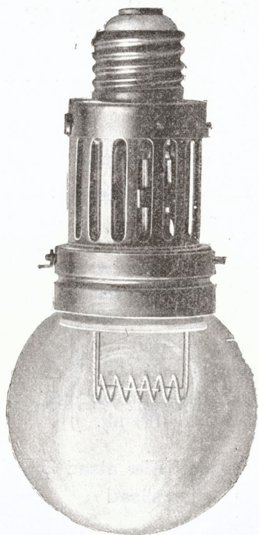
Fig. 2 NERNSTLAMP A Modell B
