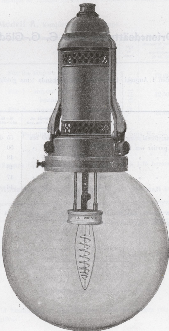
Fig. 1 NERNSTLAMP Modell A.
