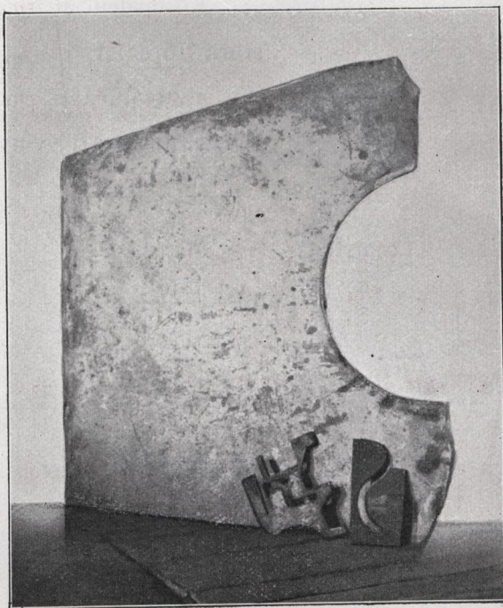
Formplåt, stansad i stansmaskin, försedd med Curvstans-anordning Efter fotografi.
