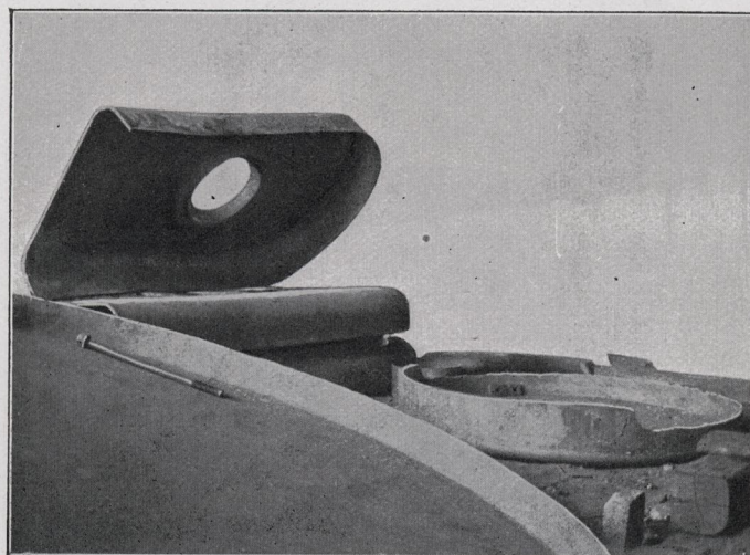
Pressade panngaflar, hvars flänskanter efter pressningen blifvit i med Curvstansanordning försedd stansmaskin bearbetade. Efter fotografi.
