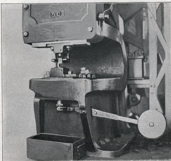
Curvstansanordning efter fotografi, till höger ligga uppstaplade stansaffall, stansade ur 40 mm. tjocka martinstålplåtar.
