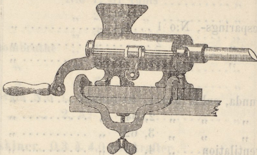
Köttskäringsmaschin.
