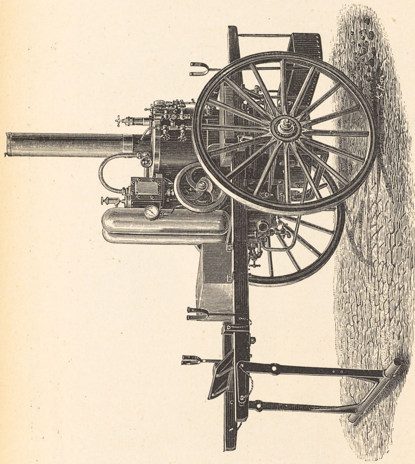
Tvåhjulig "Ludwigsbergs"-ångspruta — Granells patent — uppställd till tjänstgöring, Ludwigsbergs Werkstads-Aktiebolag, Stockholm.
