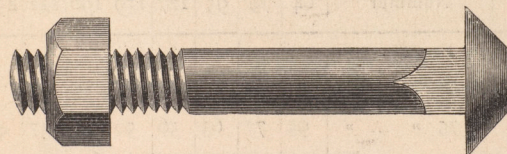
Lågt koniskt hufvud och 4-kant.
