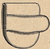
164. Tömmhållare.
