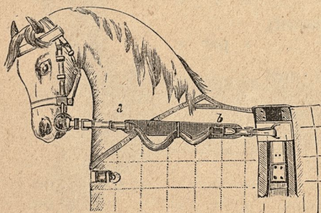
148. Gummityglar.
