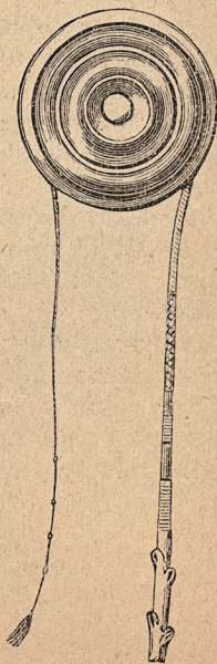
185. Piskhängare.
