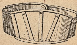
166. Ridkorsett.
