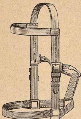
30. Grimma.
