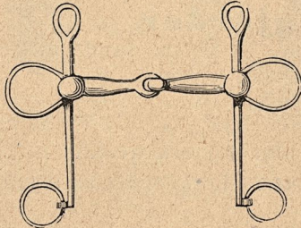
49. Vanlig Pelhamstång.
