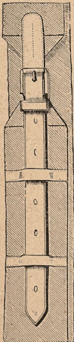
10. Öfvergjord.
