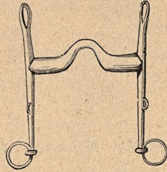
41. Vanlig ridstång.
