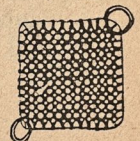
99. Polermatta.
