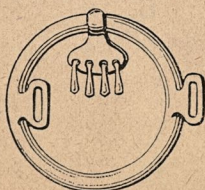
60. Fölbett.
