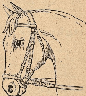
27. Grimmtrens.
