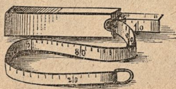
169. Hästmåttband.
