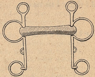
66. Gummi Pelhamstång.
