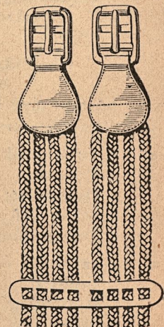
9. Lintrådgjord.
