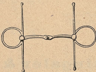
51. Vanligt trensbett.
