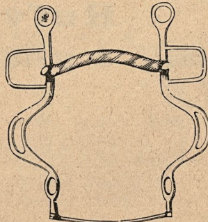
48. Parad-Kөрstång.
