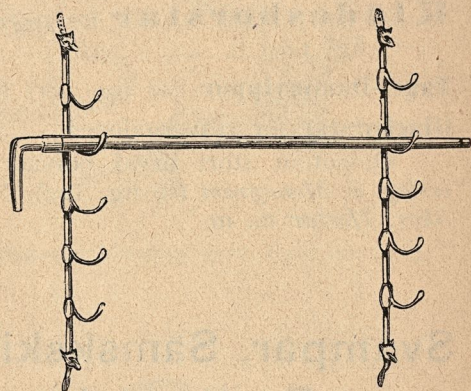
167. Ridspöhängare.
