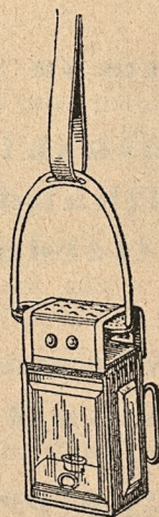
168. Stigbygellykta.
