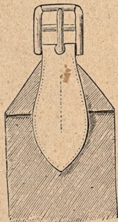
6. Yllegjord.
