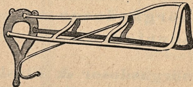
175. Damsadelhängare.
