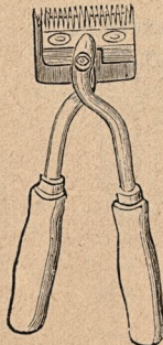
104. Hästsax.
