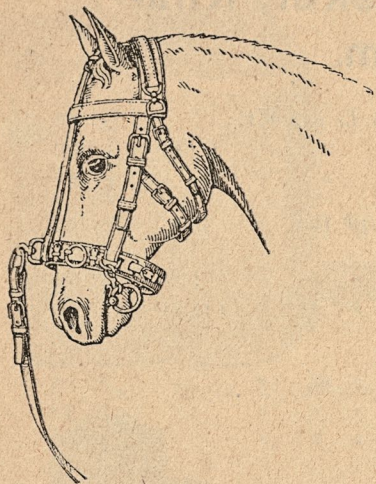
146. Kapson.
