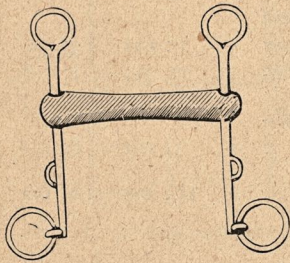
65. Gummi Ridstång.
