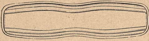
38. Däckelschabrak.
