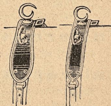
36. Däcklar.
