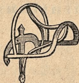
179. Kollerhängare.
