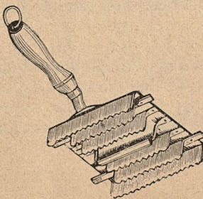
116. Ryktskrapa.
