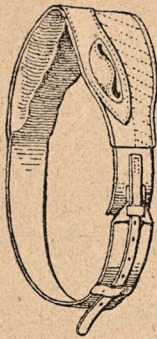
11. Förläggsgjord.
