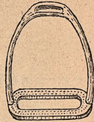
14. Herrstygbygel.
