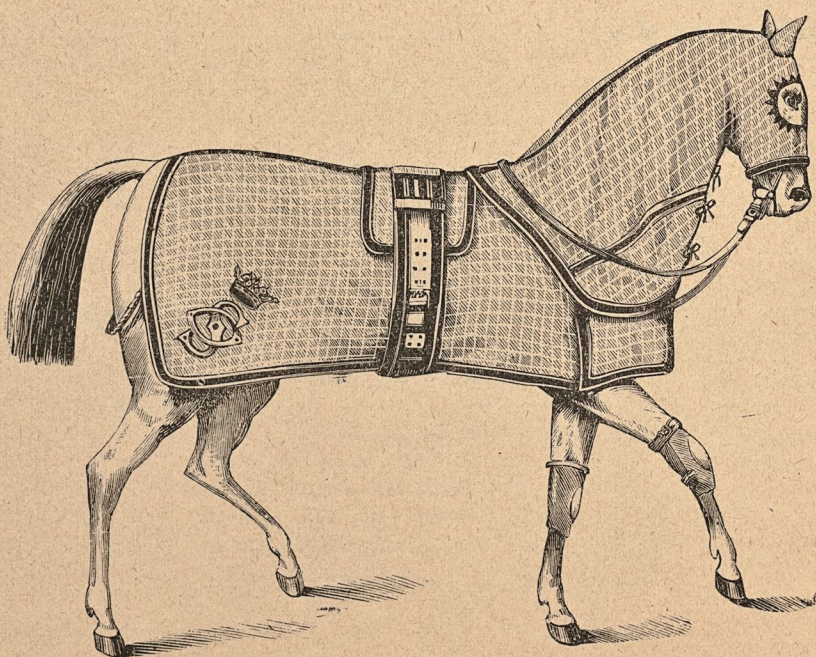
21. Täckgarnityr.
