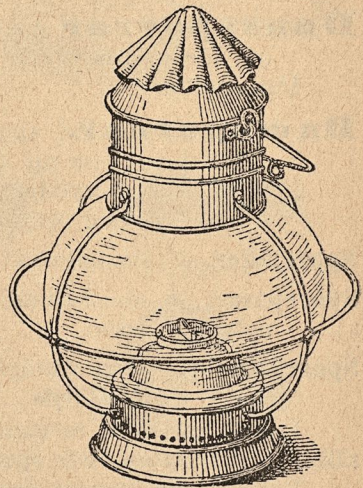
130. Stallykta.
