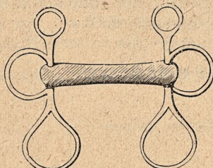
67. Gummi Körstång.
