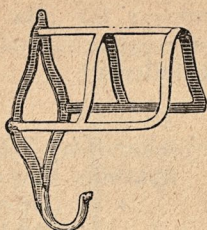
181. Enbetsdäckel- hängare.
