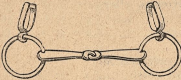
64. Ungersk Körbridong.
