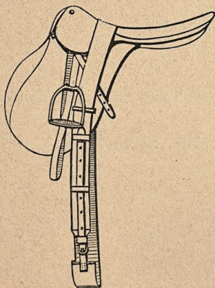
3. Slatöppningssadel.
