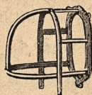
184. Körbetselhängare.
