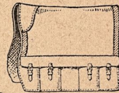
19. Kapplöpaingsvojlock.
