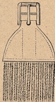
8. Snörgjord.
