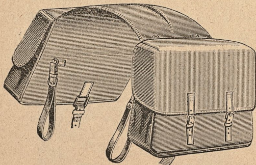
142. Stora läderpackfickor.
