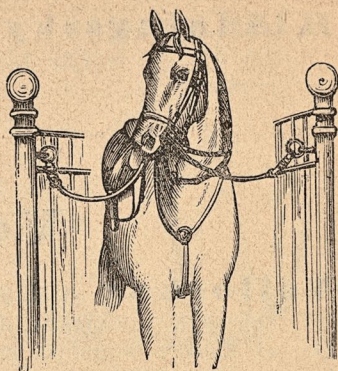
33. Omvändstyglar.
