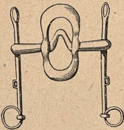
45. Tungstickarestång.
