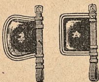
35. Skyggglappar.
