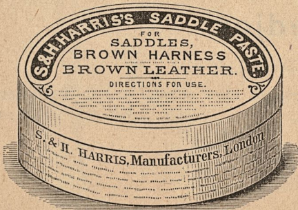
131. Sadelsåpa.
