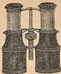
190. Kikare.
