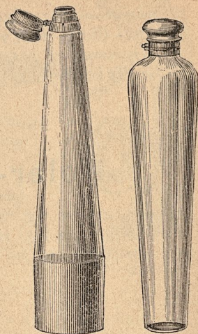
137. Sadelflaska. 138. Sadelflaska.
