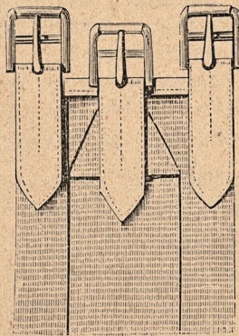
7. Fitzwilliamsgjord.
