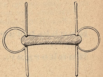
68. Gummi Trensbett.
