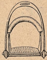
16. Damsäkerhetsstygbygel.
