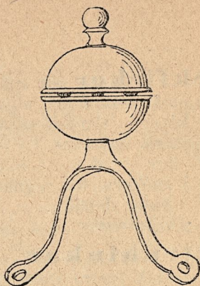
173. Klockspel.
