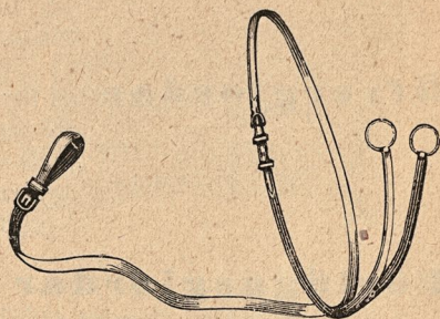
28. Martingal.
