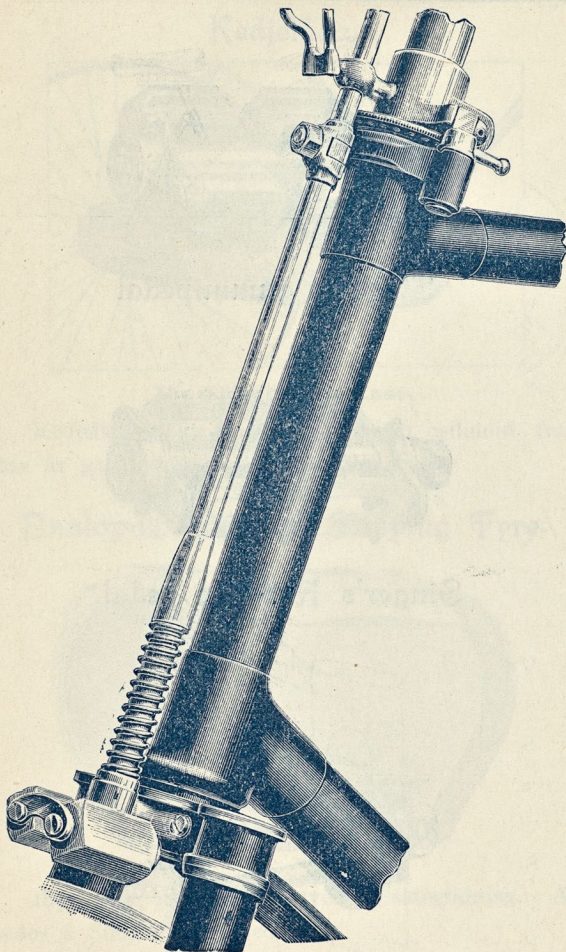
Singer's kulstyrning och patenterade styrstångslås. Hall's patenterade gummbroms.
