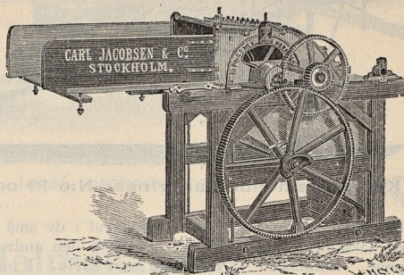
Köpings Stifttröskverk N:o 3 och N:o 6 med hufvudaxeln nedflyttad i de nedre lagren för direkt tillkoppling till vandring.
