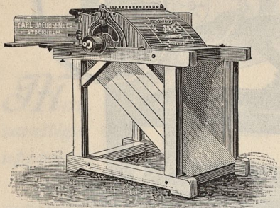
Köpings Stiftröskverk N:o 1 och N:o 5 med remskifva.
