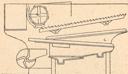
Genomskärrning af 3 och 4 hästars tröska.
