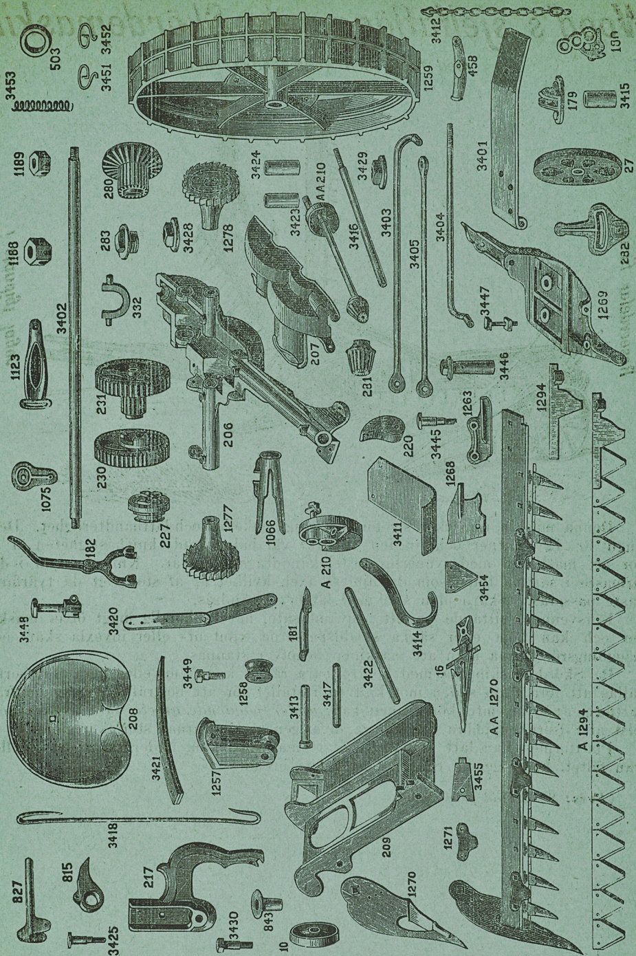
Reservdelar till Walter A. Wood's nya Slättermaskin.
