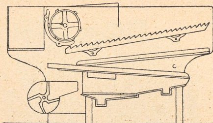
Genomskärning af 3 och 4 hästars tröska.
