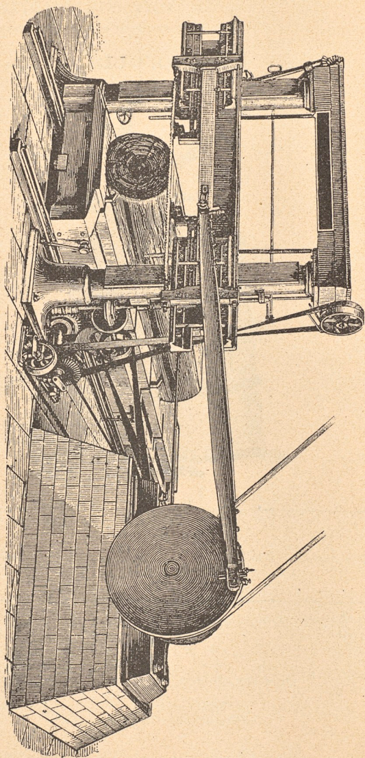
Horizontal Stocksåg för Löffträd.
