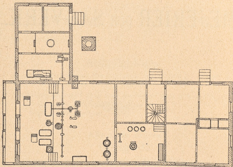
Andelsmejeri för 8 à 10,000 liter mjölk pr dag.
