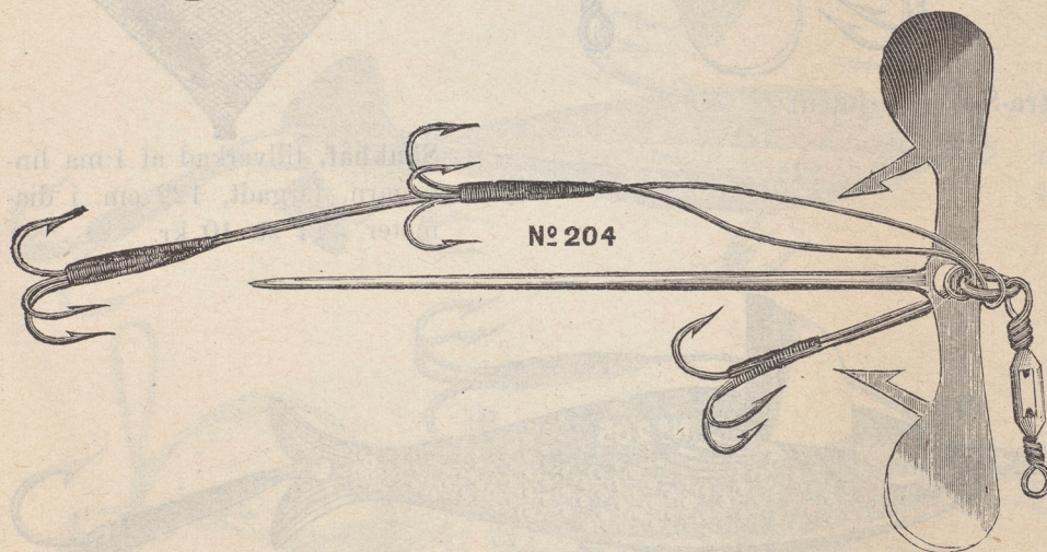
N:o 204. Non-Plus-Ultra-Swivel (öppen), längd c. 8½ cm., med stång och propeller, afsedd att dervid fästa ett naturligt bete. Denna swivel är ny och af alldeles utmärkt beskaffenhet. Pr st. 1,35.
