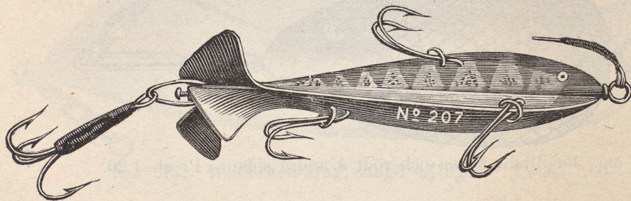
N:o 207. Turbin-Swivel, längd c. 8 cm., målad i flera färger, ny sort och af utmärkt beskaftenhet. Pr st. 2,25.
