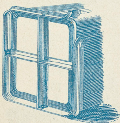
Flaskans botten med utvikt bottenband sedd underifrån.
