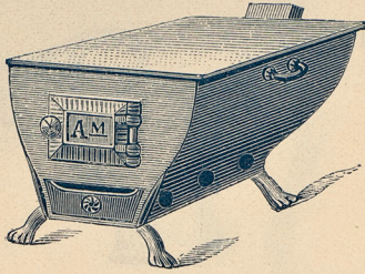
Strykugnar, med flat häll.
