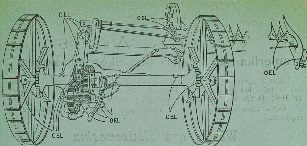
Maskinen sedd bakifrån.
