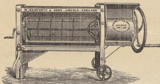
Klass I med ställbar Cylinder.
