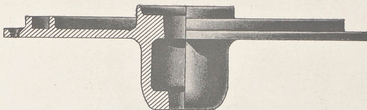
Bottenstycke.
