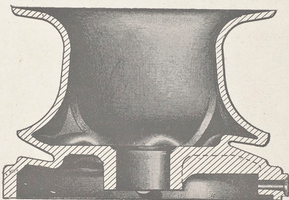
Varpklamp.
