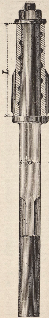
Sätshärdade, med väl påpassade bössor, muttrar och försticklar.
