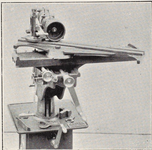
Slipning af giggar.
