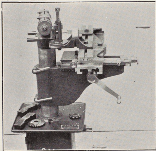
Fasonslipling efter ledare.
