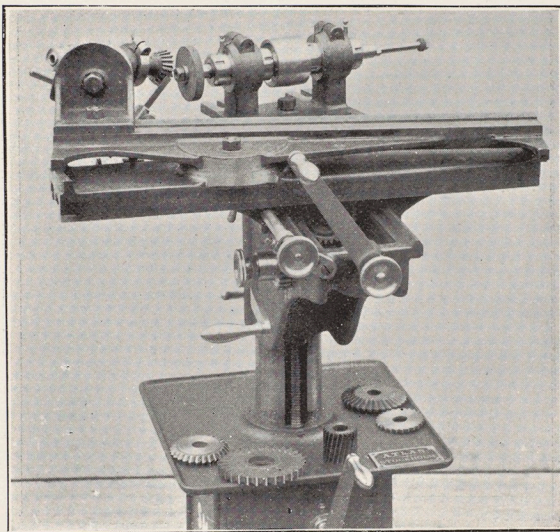
Skärpning af frästrissor.
