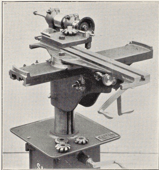
Skärpning af frästrissor.
