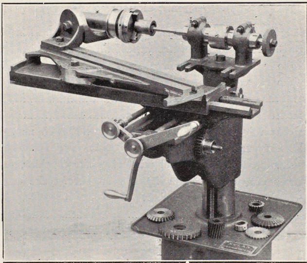
Slipning af cylindriska & koniska håål.
