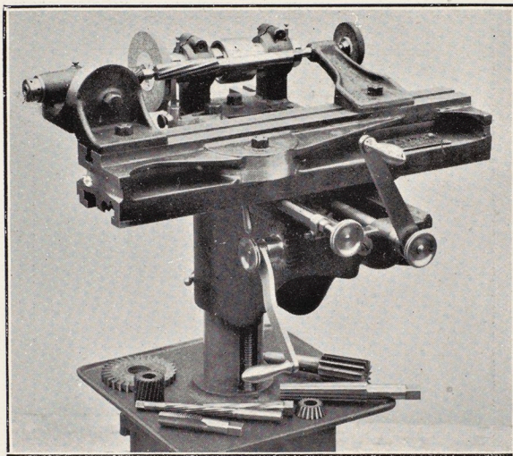
Skärpning af brotchar. & fräsar.
