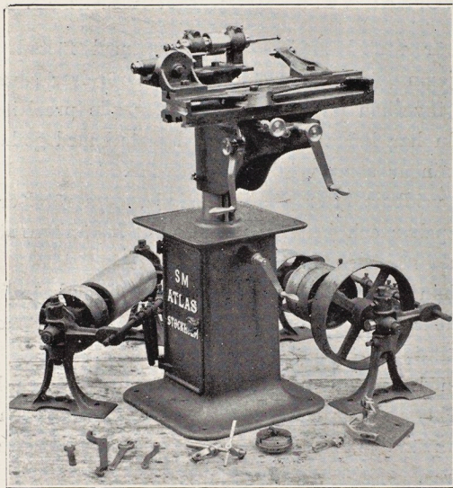
Universal Verktögs-Slipmaskin S. M.
