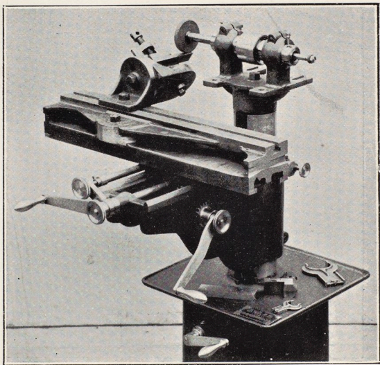
Slipning af sned yta.
