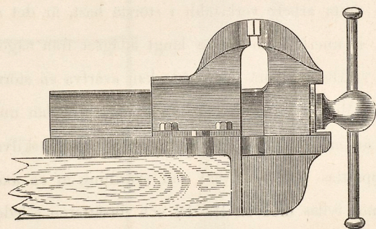
Gjutna Paralell-skrufst d med fastskruvade st l- k ftar.
