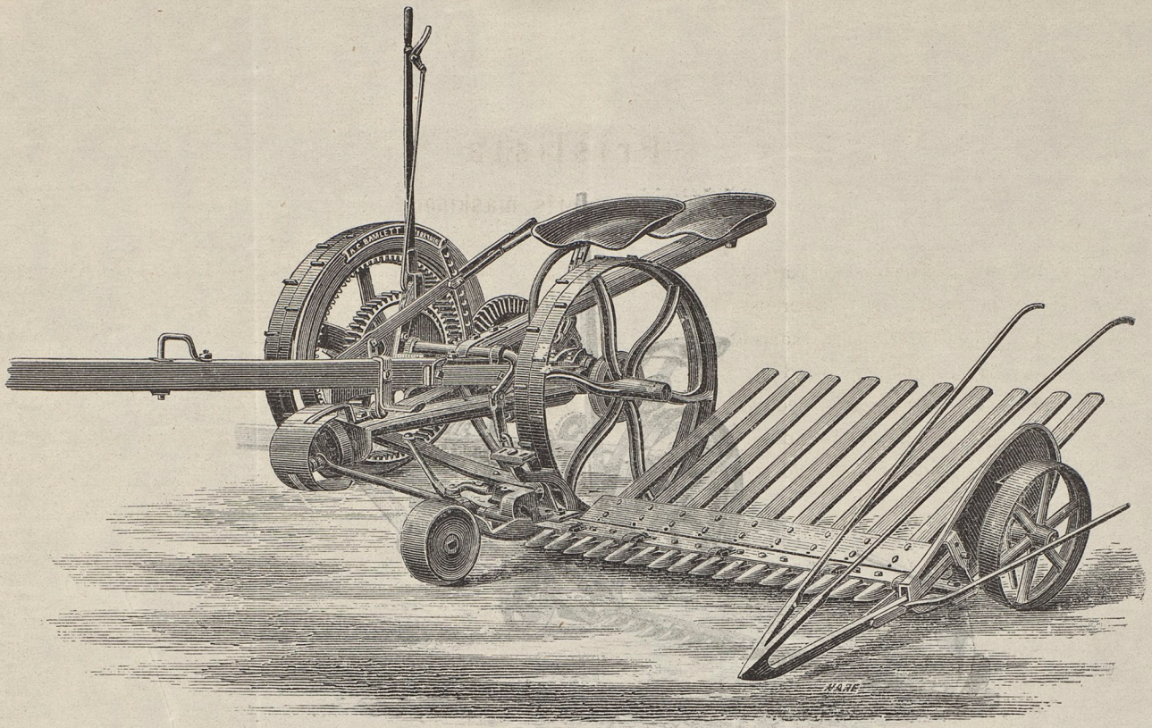
BAMLETTS MASKIN N:o 4.
