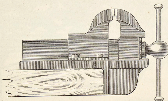
Gjutna Parallel-Skrufstäd med fastskrufvade stälkäftar.
