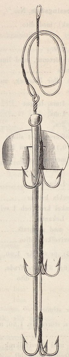
Fig. 3. Spjutsvivel.
