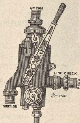
Modell för storlekarne N:o 3 och högre.
