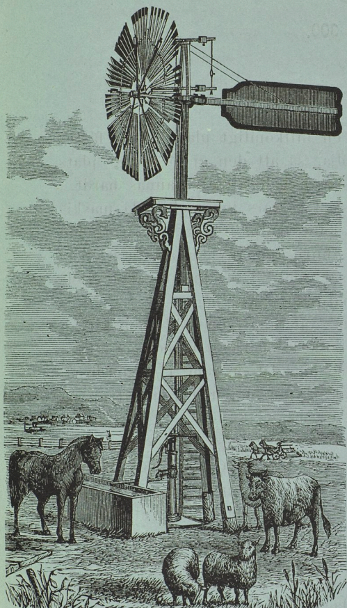
Figuren utvisar maskinen apterad för pumpning af vatten.
