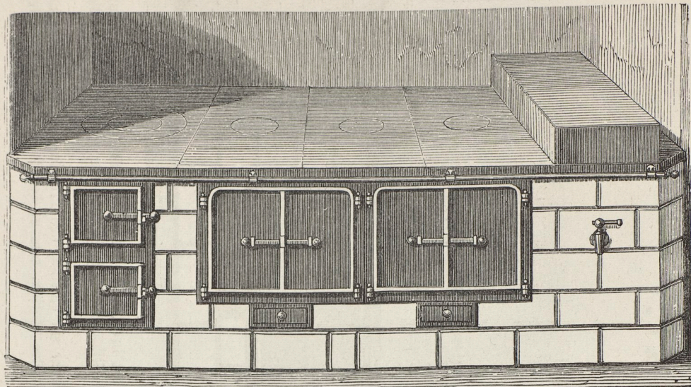
Hällen 8.30 fot lång, 3.67 fot bred. 2:ne stekugnar, hvardera 1.87 fot bred, 1.20 fot hög, 3.08 fot djup. Vattenreservoir af koppar med tillhörande metallkran.
