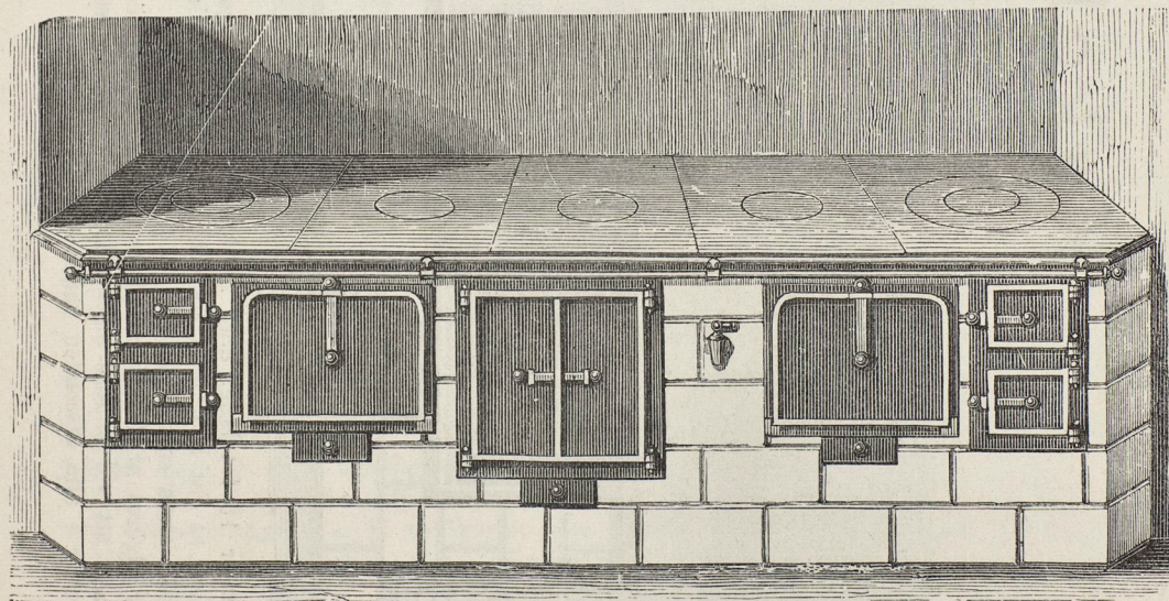
Hällen 9 fot lång, 2.67 fot bred. 2:ne stekugnar, hvardera 1.40 fot bred, 1.00 fot hög, 2.50 fot djup. 1 varmuugn. Vattenreservoir af koppar jemte metallkran. Denna spis är äfven fördelad i 2:ne olika stora spisar med hvar sin eldstad, hvilka äro oberoende af hvarandra i likhet med Litt. A., så att matlagning för mindre behof kan verkställas i endast en spis, om så önskas.
