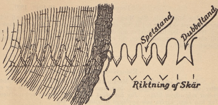
Fig. 5. Skiss af tandningen å sågbladen. (Amerikansk Tandning.)
