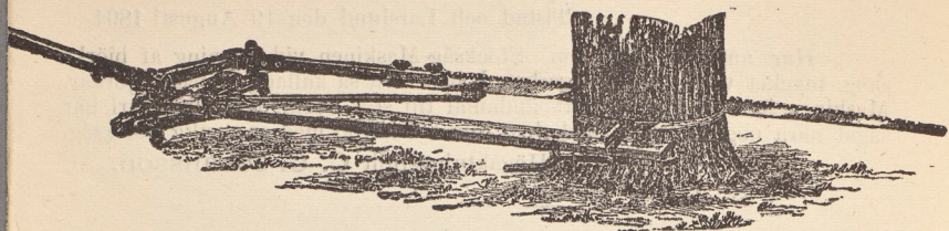
Fig. 2. I läge för fällning.
