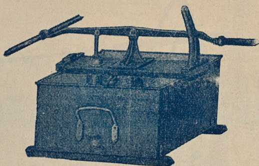
Fig. 3. Enkelverkande med Kar af jern.
