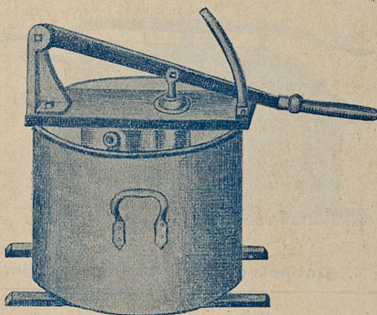
Fig. 2. Enkelverkande Kar af jern.
