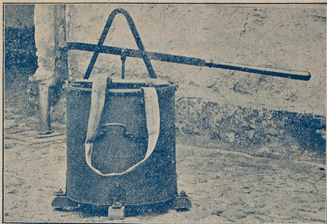
Fig. 1. Enkelverkande Kar af jern.
