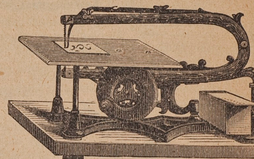
* Hand-Löfsågningsmaskin N:o 3. Sågvidd 40 centimeter. Denna maskin liknar fullkomligt N:o 2, undantagandes, att den är försedd med fotställning, hvarigenom den ej behöfver fastskrufvas; dessutom arbetar den stadigare. Kan ej drifvas med tramp. Pris med ett dussin sågblad, 2 borrar, skrufmejsel, oljekanna och verktygslåda, Kr. 20. Inrättning för bortblåsning af sågspån Kr. 6.
