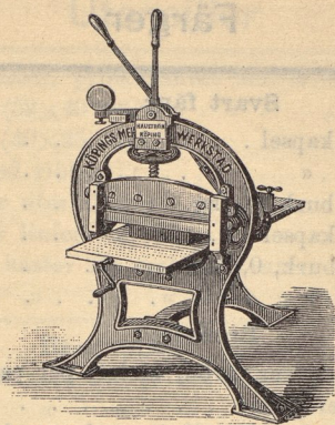
Pappersskärmaskin N:o 2.
