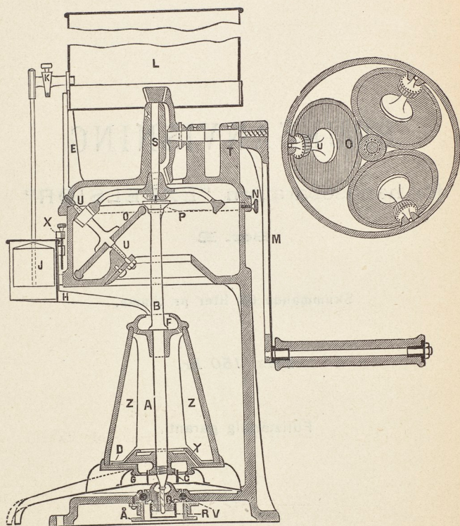
Genomskärning af Excelsiorseparatorn.
