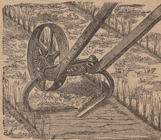
•Planet jr.• Enhjulig Hacka skyfflar mellan raderna.
