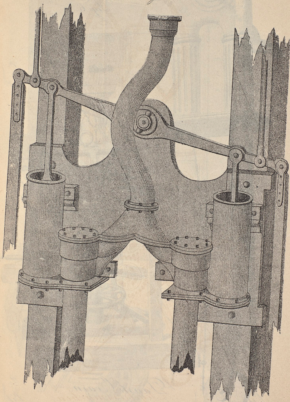
Große Pumpwerk.
