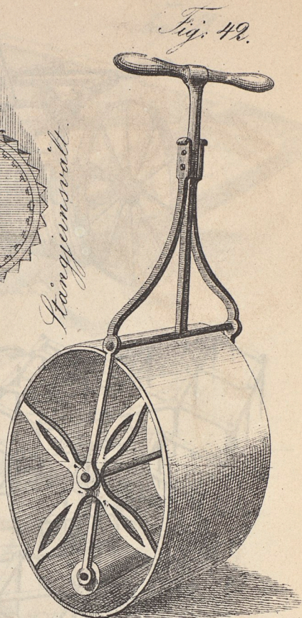
Trädgårds-Vält.
