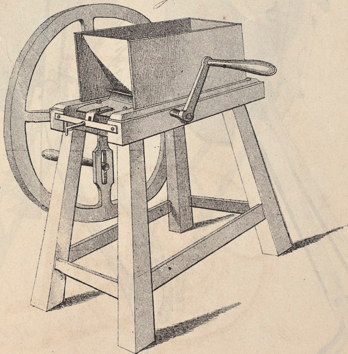
Gröpmalningsmaskin.
