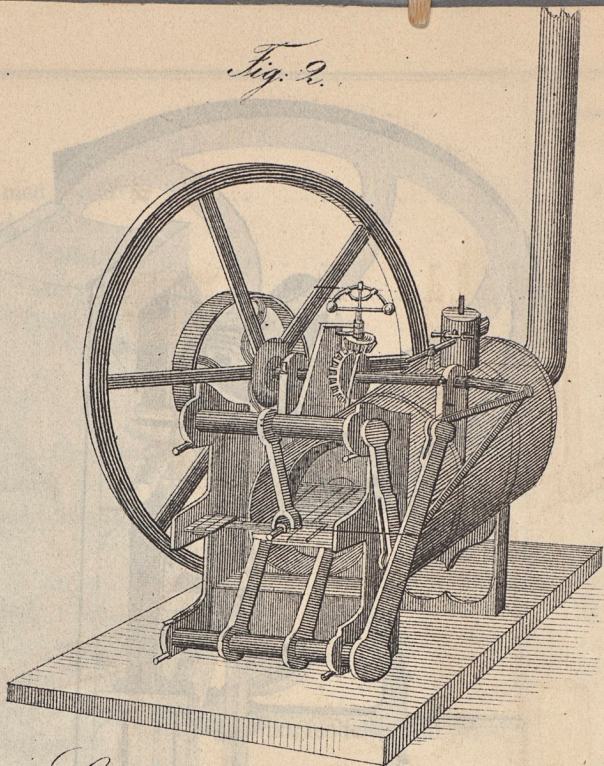
Calorikmachin.
