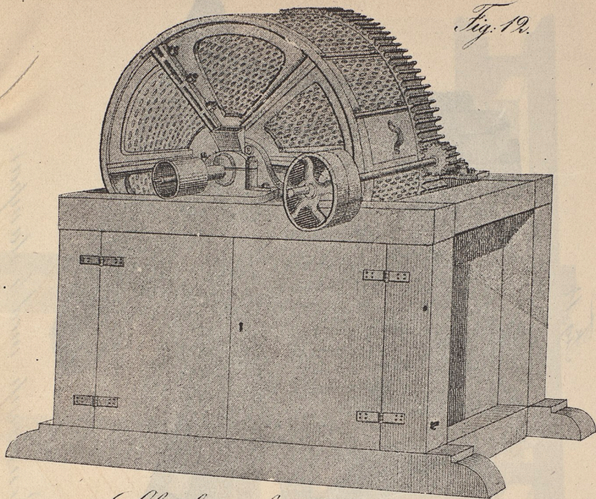
Skalmachin.
