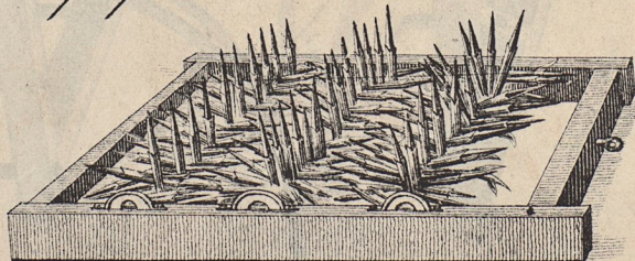
Rullharf med 3 re Axlar och pinnar af smält jern.
