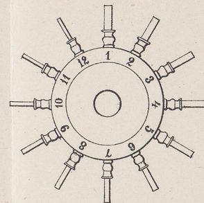
Mått för nyckelrör.
