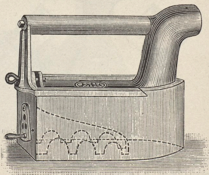
S. k. Ång-pressjern för skräddare (att elda med kol).
