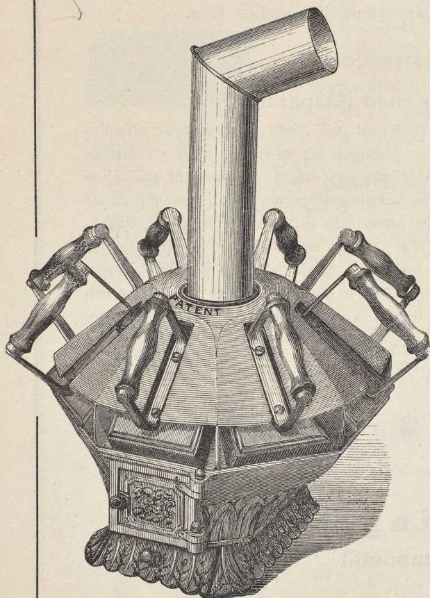
Strykjernskupor att anbringas på spisar med plats för 6 jern.
