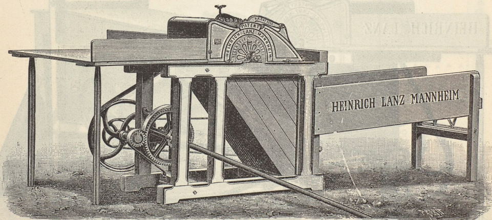
2 hästars tröskverk till längloge.
