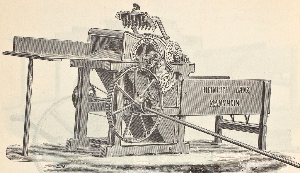
Ny patenterad handtröska uppställd till hästvandring. Pris 160 Kr.
