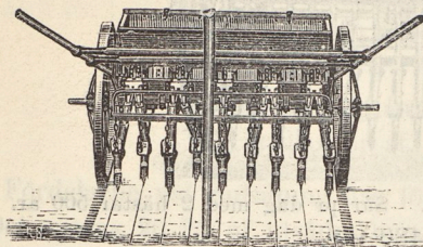
1 meter Radsåningsmaskin 9 rader.
