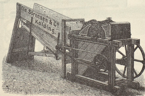
Handtröska med halmrystare och 2 säll. Pris 250 Kr.
