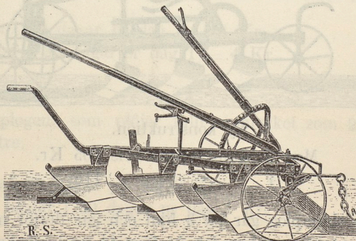
Normal trefärig plog, ny konstruktion.
