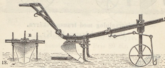
Universalplogen som drillplog med breda rader.
