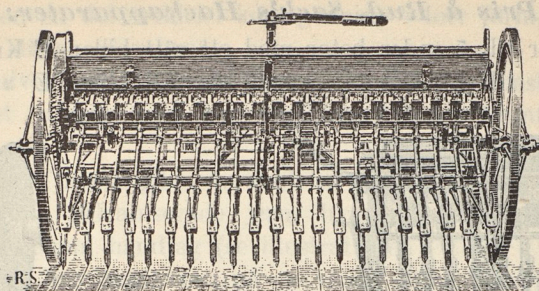
2 meter Radsåningsmaskin; 21 rader. Sår pr dag med 2 hästar 500 ar. Pris Kr. 480 —
