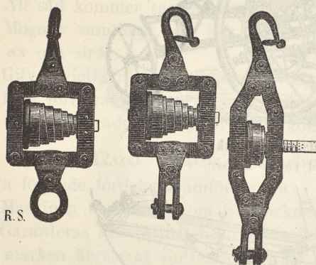
Elastiskt fjederdrag. som medföljer radsåningsmaskinen. Extra pr st. Kr. 12.
