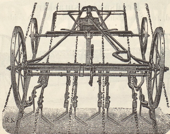
2 meter Radsåningsmaskin uppställd till rensning af 4 rader betor.
