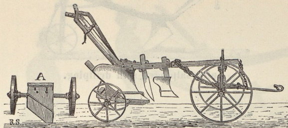
Universalplog med transportkärra. Pris för kärran 12 Kr,
