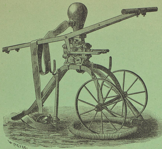
Dubbelverkande Spruta N:o 2.
